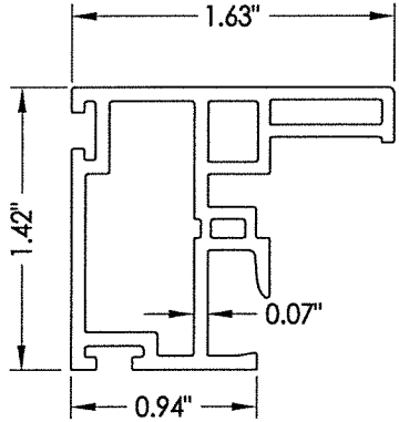
4 STILE
